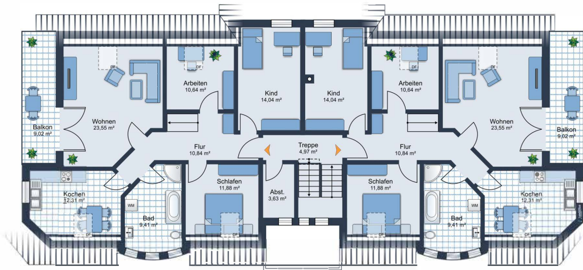
Obergeschoss
